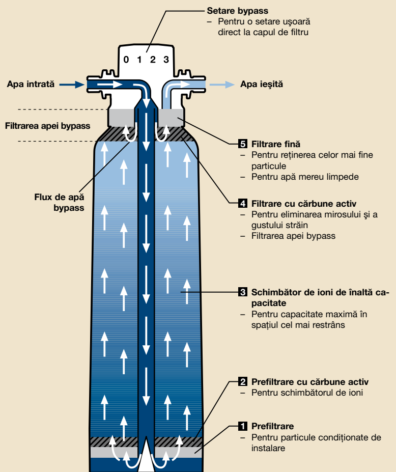
Structura unui cartuș filtrant BWT bestmax-PREMIUM cu filtrare cu 5 trepte
